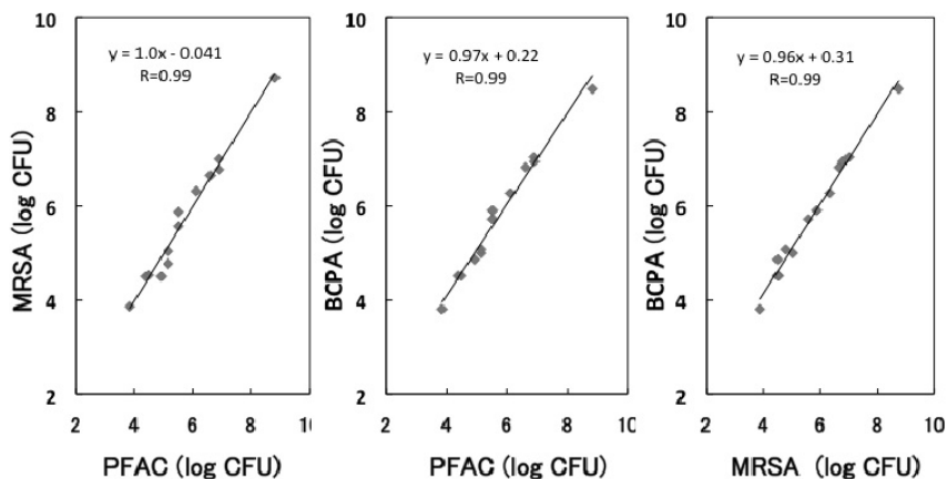
図3. 異なる培地で測定した肉類の乳酸菌生菌数の相関性
