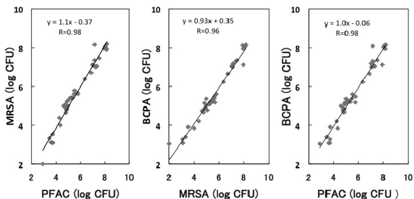
図1. 異なる培地で測定した漬け物中の乳酸菌生菌数の相関性
