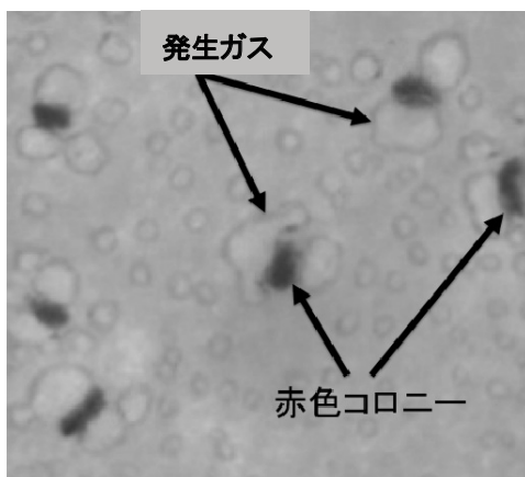
図2. PFACで観察されるガス産生菌
